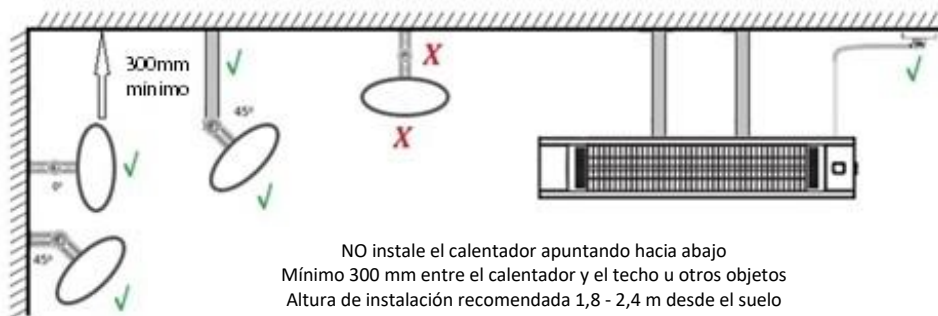
Diagrama 2: Posición de montaje en la pared / techo
