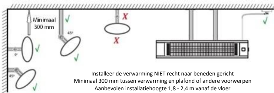
Diagram 2: Correcte positive wand / plafond
